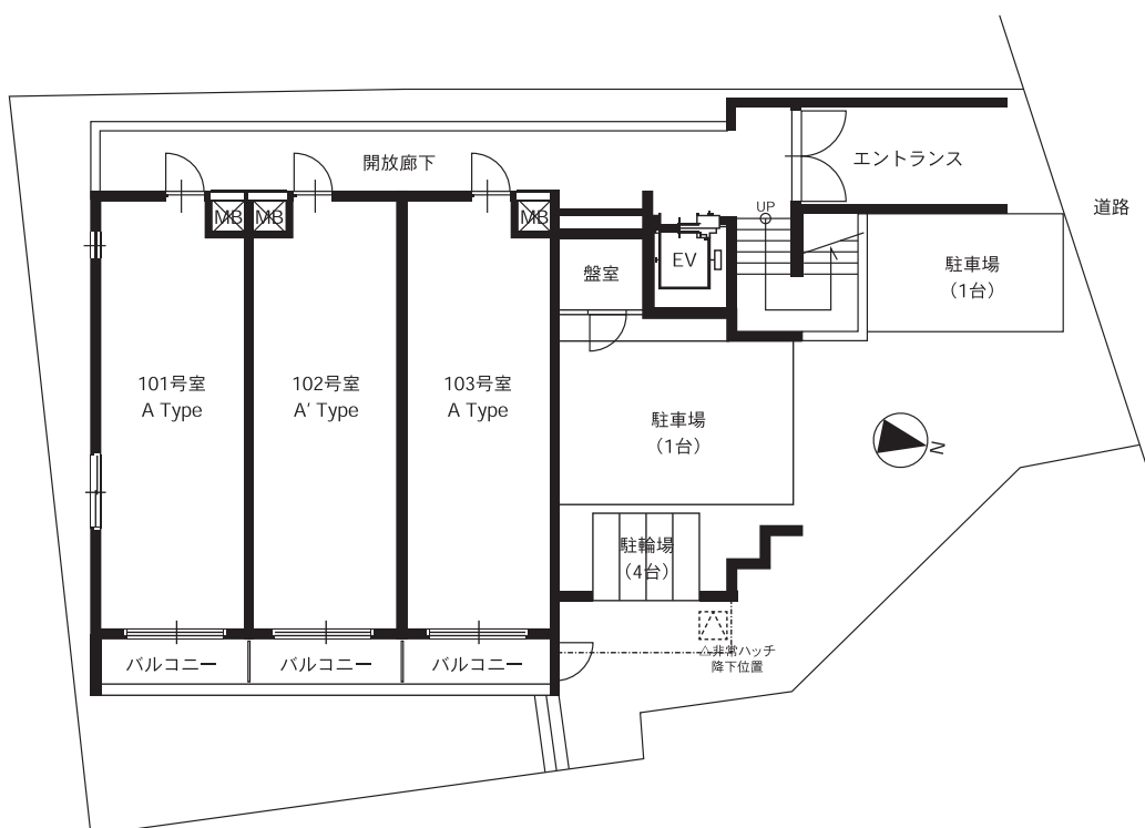
1階平面図
